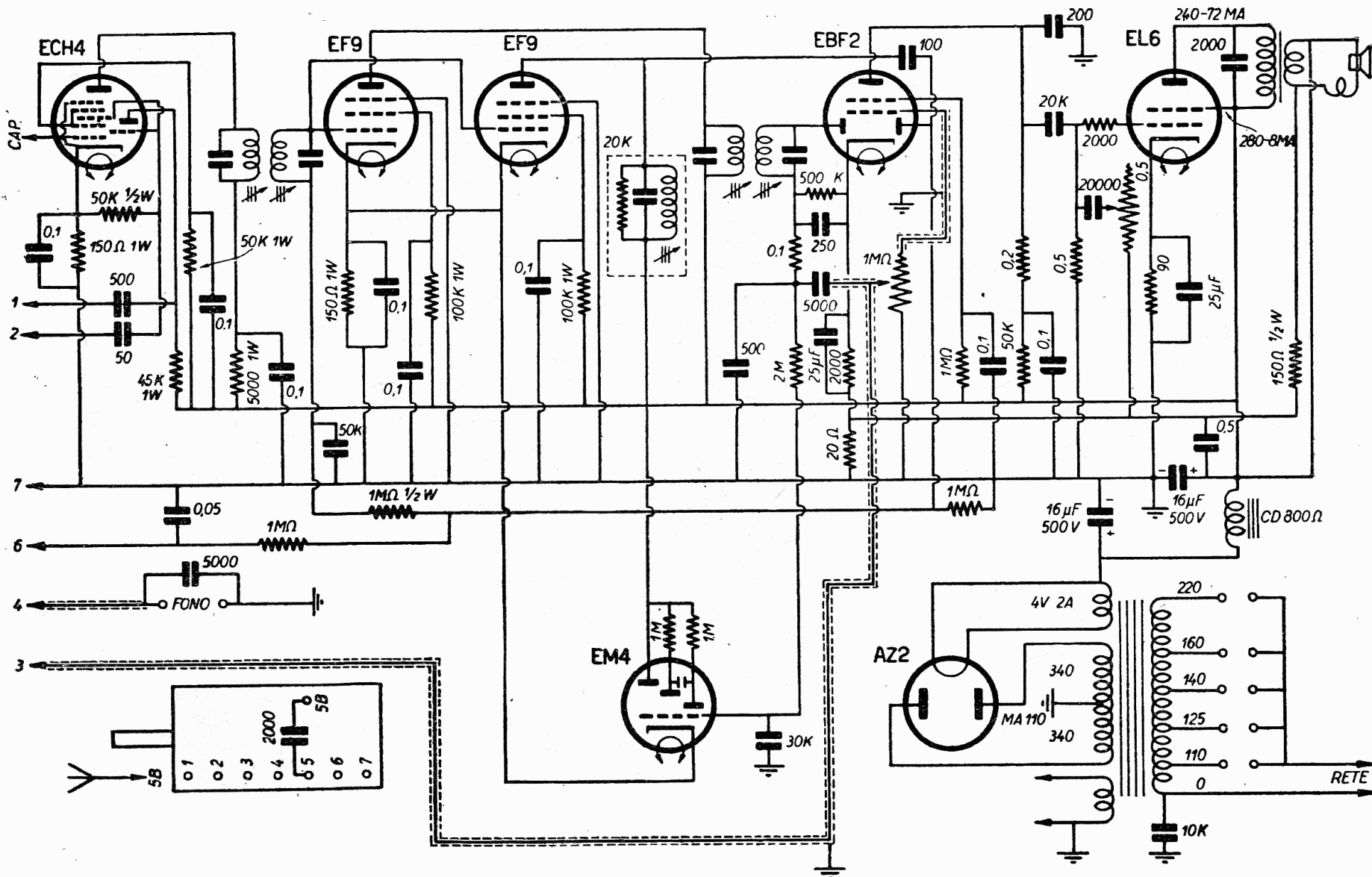
LIAR - Mod. 658. Supereterodina a 5 valvole, più una EF9 per l'amplificazione del CAV, e una EM4 indicatrice di sintonia. Media frequenza: 465 kc/s. C.d.t. bobina campo: 88 V. Prod. 1947-48. (Gruppo AF a permeabilità NOVA P1).
